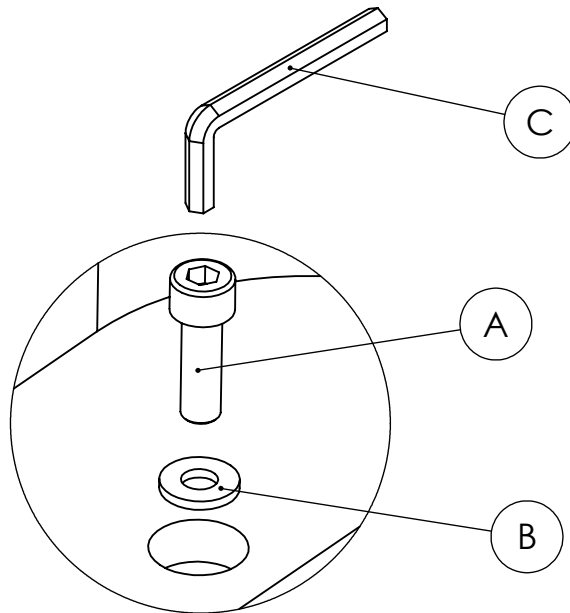
DETALJ A
